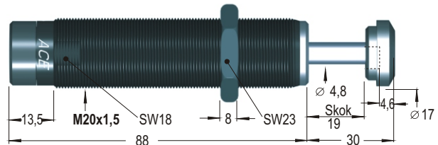
MA 900 M
