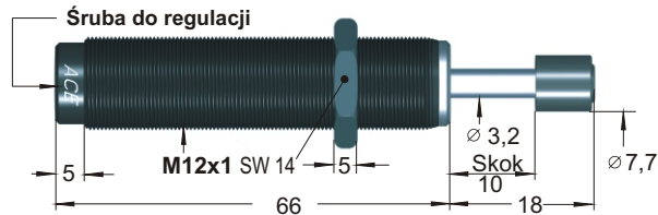
MA 50 M-B
