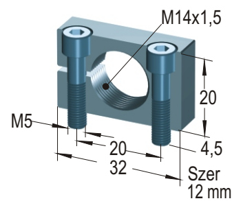
kołnierz zaciskowy
