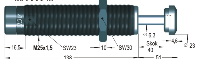
MA 900 M
