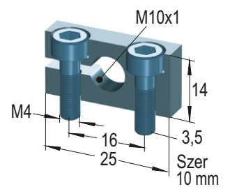
kołnierz zaciskowy
