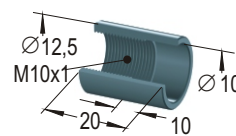
tuleja zderzaka
