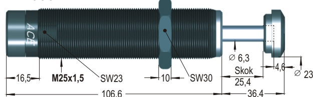
MA 600 M
