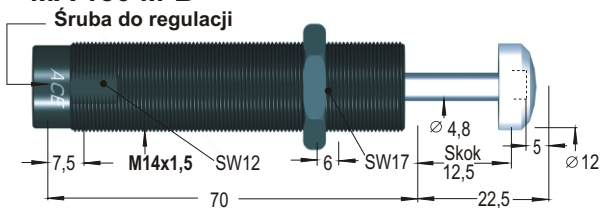
MA 150 M-B
