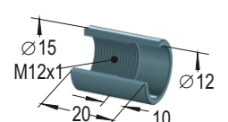
tuleja zderzaka
