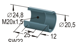
tuleja zderzaka
