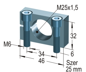
kołnierz zaciskowy
