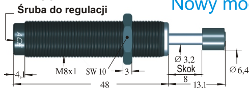
MA 150 M-B
