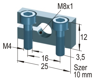
kołnierz zaciskowy
